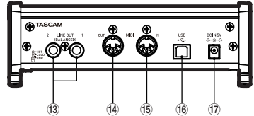
Panel trasero del US-2x2
