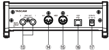
Face arrière de l'US-2x2
