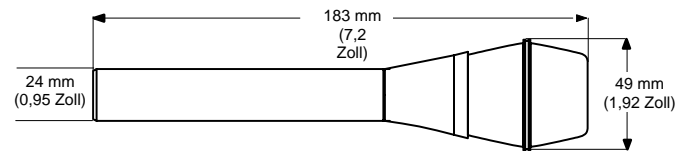
GESAMTMAßMESSUNGEN ABBILDUNG 5
