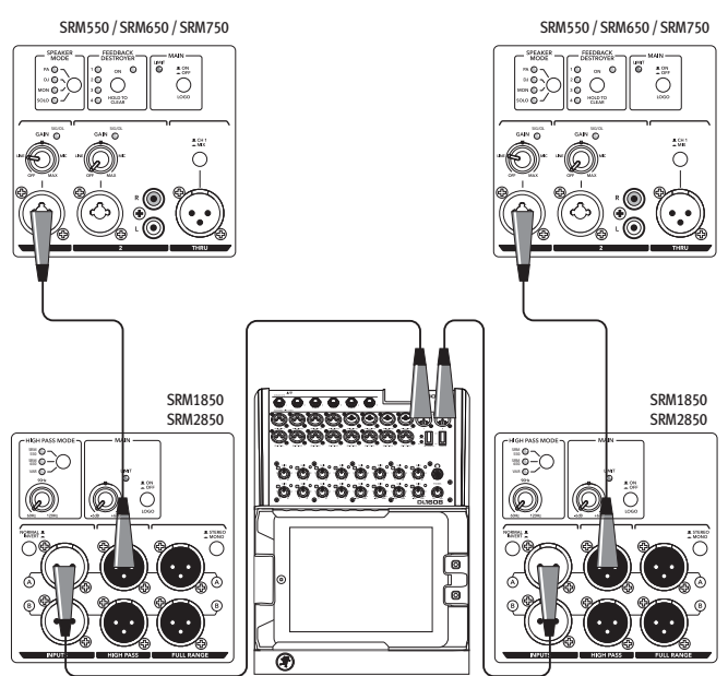
PA System with two powered subwoofers Sistema PA con dos subwoofers autoamplificados Système de sonorisation avec deux Subwoofers actifs PA-System mit zwei aktiven Subwoofern
