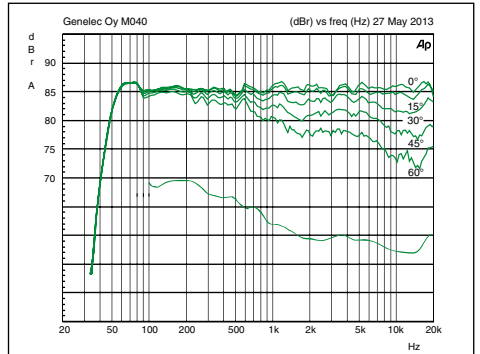
图 7. 曲线描述了M040在水平方向上的指向特性。较低的曲线描述了音箱的功率响应。
