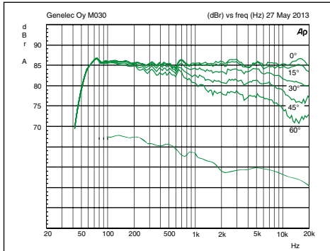
图 6. 曲线描述了M030在水平方向上的指向特性。较低的曲线描述了音箱的功率响应。
