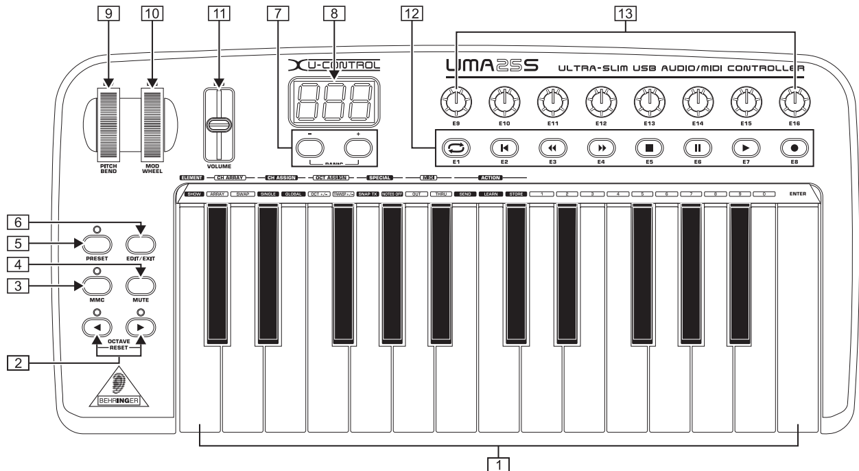
Fig. 3.1: Superficie de control del UMA25S
