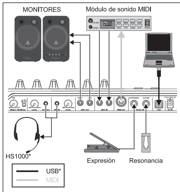
Fig. 1.3: Ejemplo de conexión
