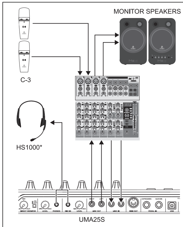
Fig. 4.1: Ejemplo de conexión usando el UMA25S
