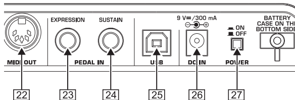
Fig. 3.3: Más conexiones en la parte trasera
