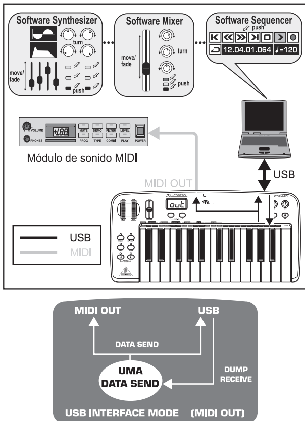
Fig. 1.3: Modo USB con MIDI OUT
