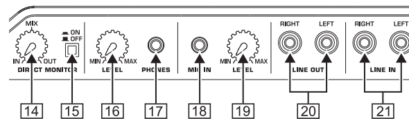
Fig. 3.2: Conexiones de audio en la parte trasera
